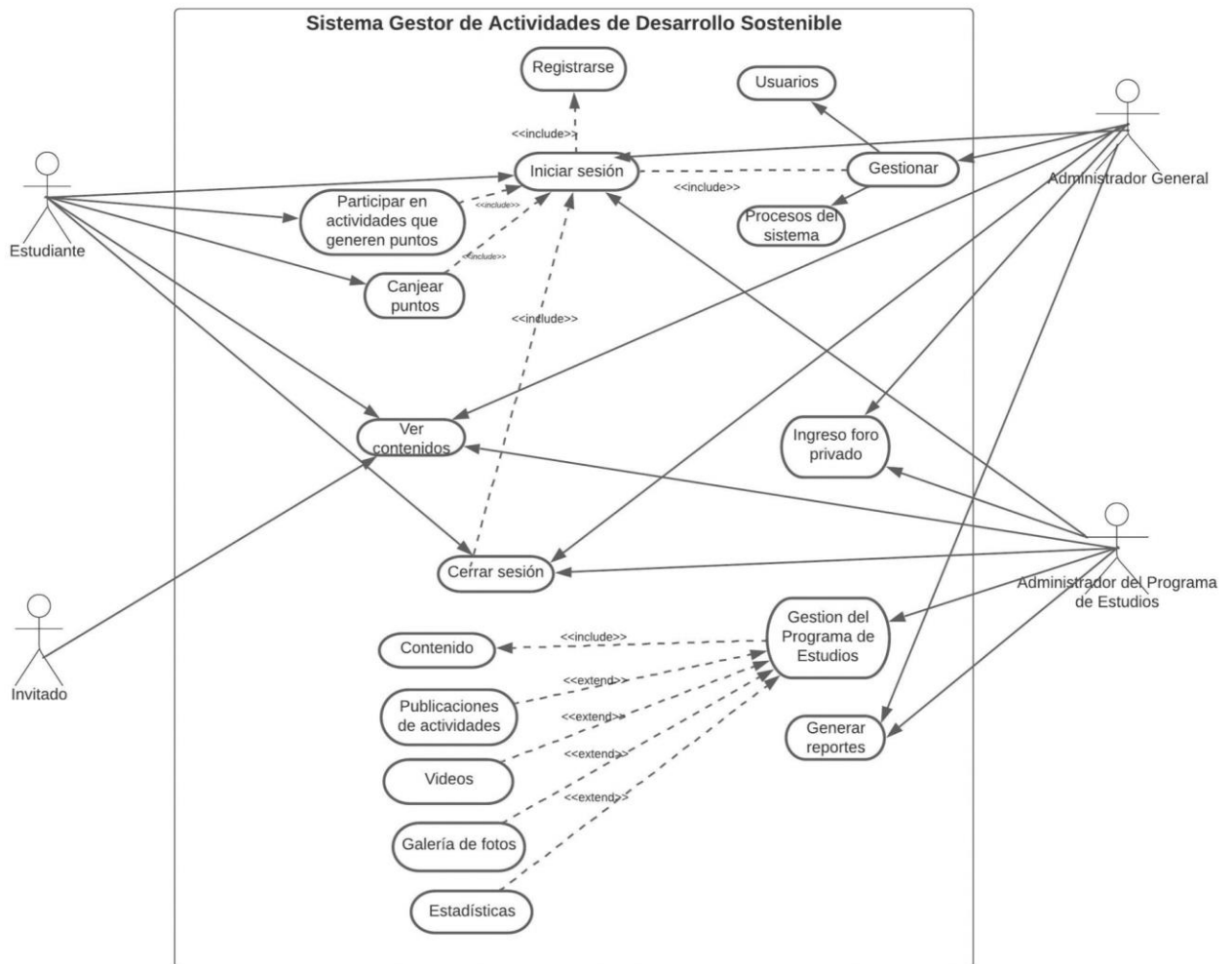
Figura 1. Diagrama de casos de uso para el Sistema Gestor de Desarrollo sostenible
